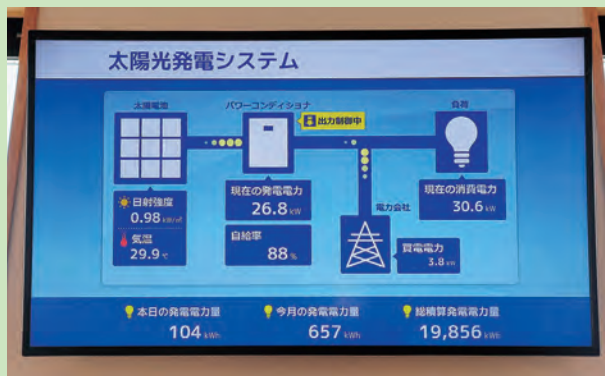
太陽光発電システム表示
